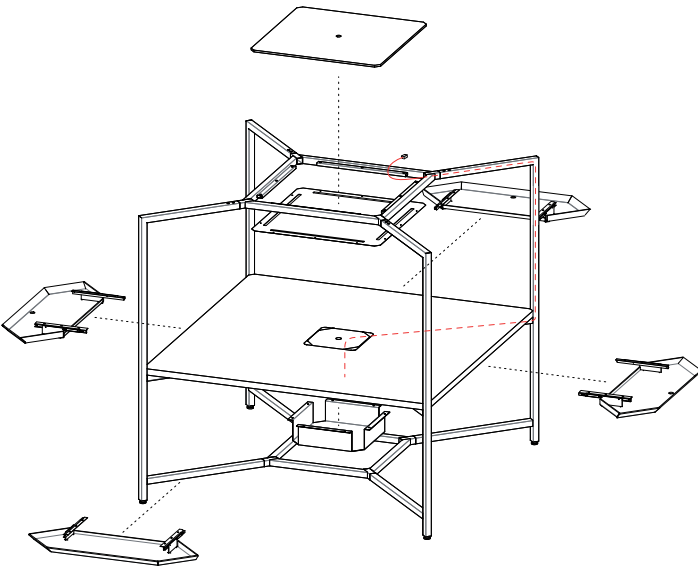
Modulo con overhead e illuminazione integrata / Module with overhead with integrated lighting / Modul mit Aufbau und integrierter Beleuchtung / Module avec arche et éclairag intégré / Módulo con cubierta con iluminación integrada
